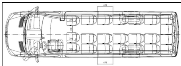
Implantation 22+1 avec porte avant droite.
