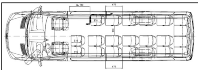
Implantation 21+1+1 avec porte latérale coulissante.
